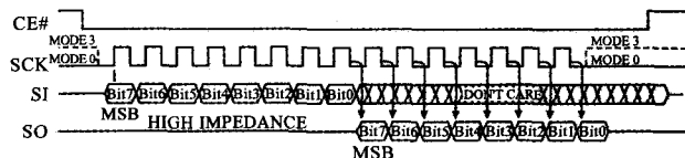
图 1 SST25VF020 的工作时序图
