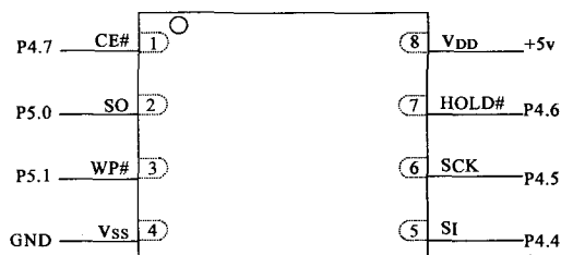
图 2 引脚连接
