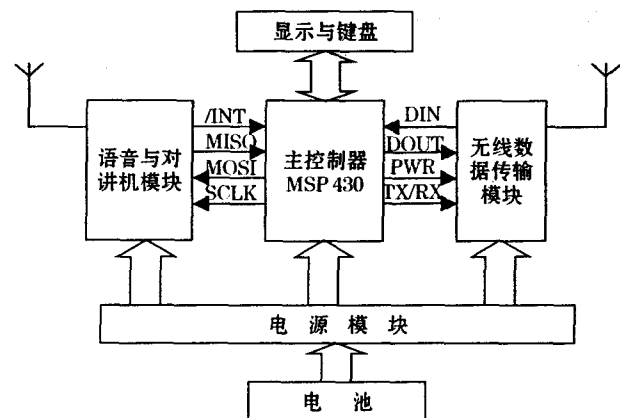
图2 报警节点组成框图
