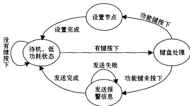
图 4 报警节点工作状态,发送部分
