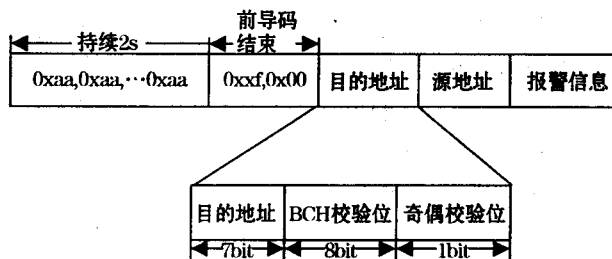
图5 一帧数据格式
