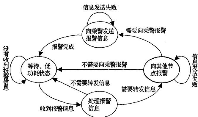
图 3 报警节点工作状态,接收部分
