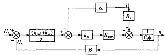
图 3 转速、电流双闭环控制原理
