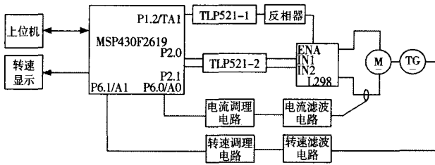
图 1 双闭环调速控制系统电路原理图
