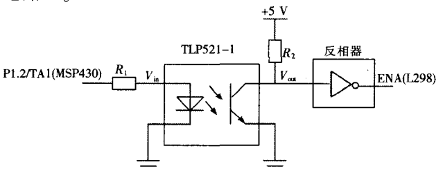
图 2 TLP521-1 实现电气隔离电路图
