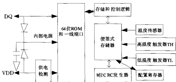
图2 DS18B20 内部结构图
