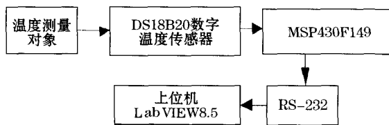
图1 系统硬件组成框图
