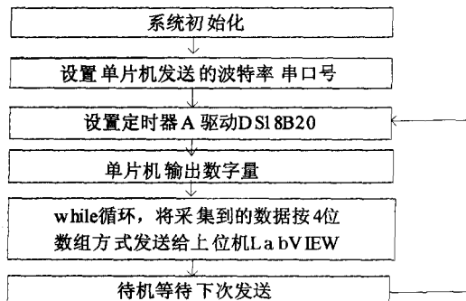
图5 MSP430F149 程序流程图
