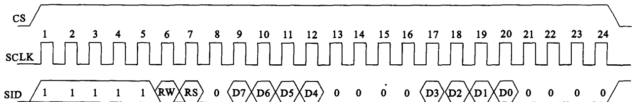
图1 串行模式下数据传输
