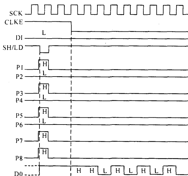
图2 74HC165时序图
