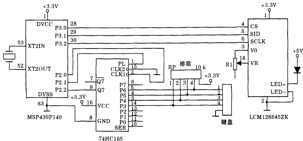
图3 LCM128645ZK,74HC165与MSP430微处理器接口电路
