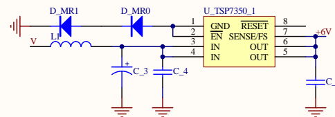
舵机稳压 +6V
