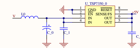
CPU稳压 +5V
