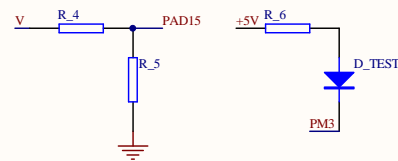
电压测量及指示电路
