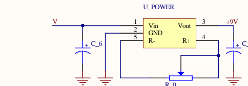
摄像头升压 +9V
