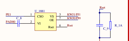
视频信号分离电路
