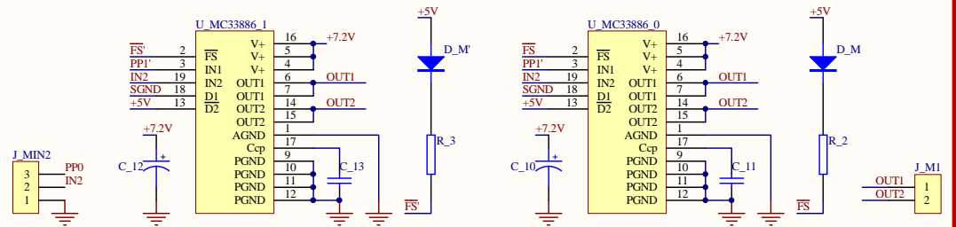
电机驱动模块
